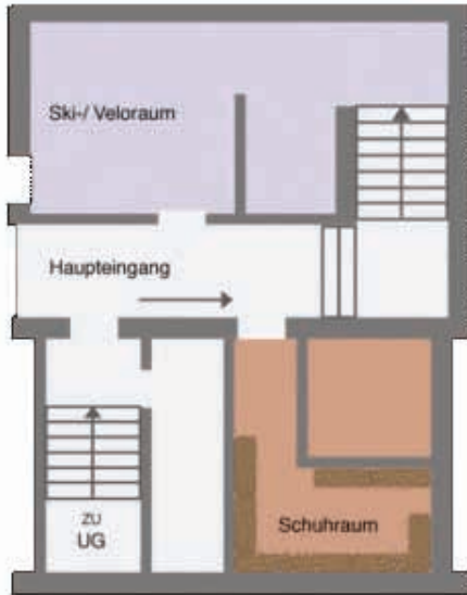
Erdgeschoss
